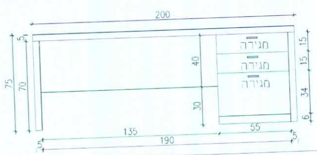
חזית - 1
