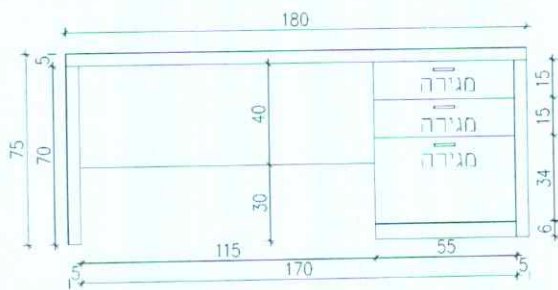
1 - חזית
