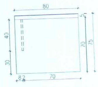
חזית - 2
